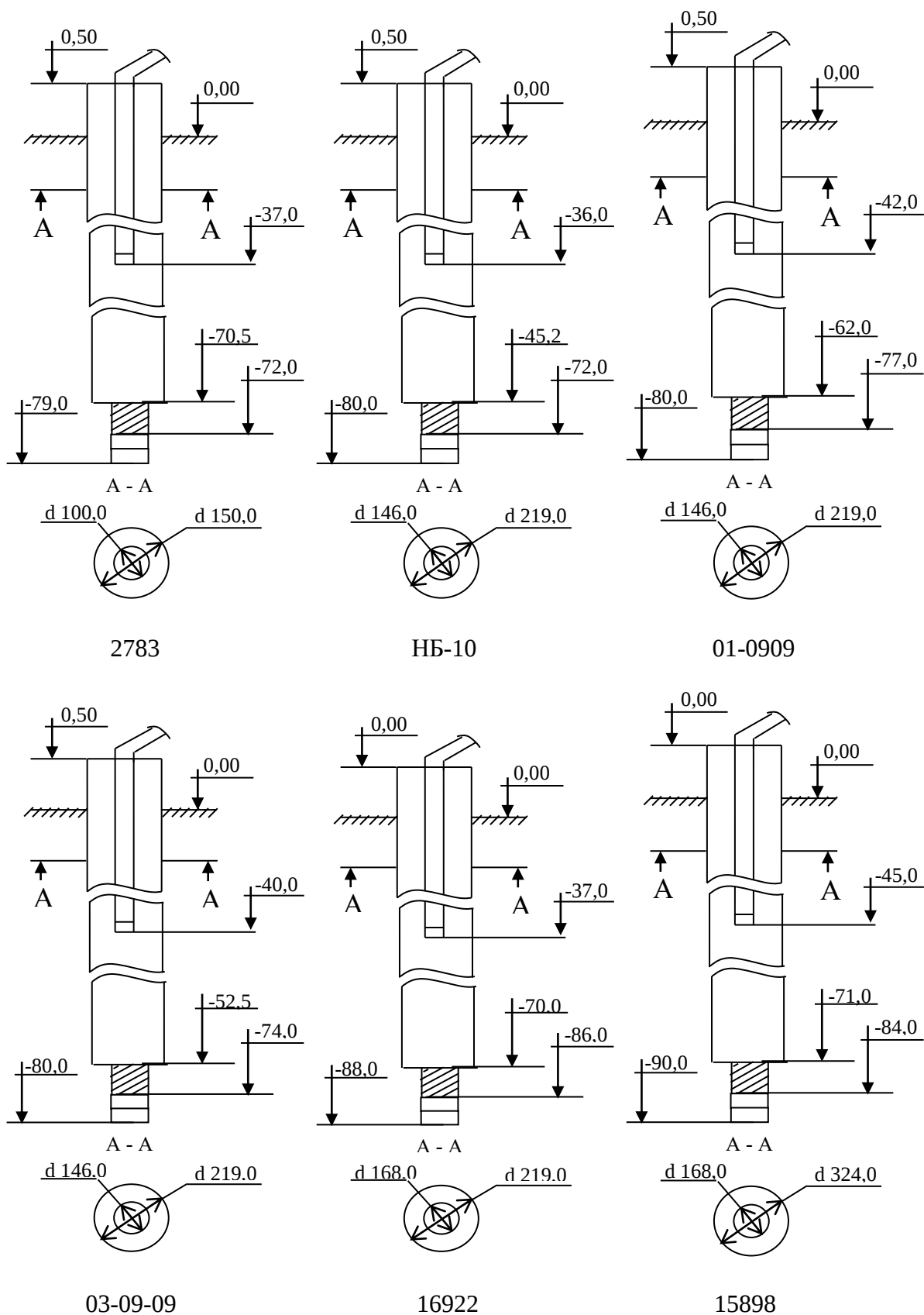
Рисунок 4 – Принципиальная схема установки водоподъемного оборудования в скважинах Ярковского сельсовета
