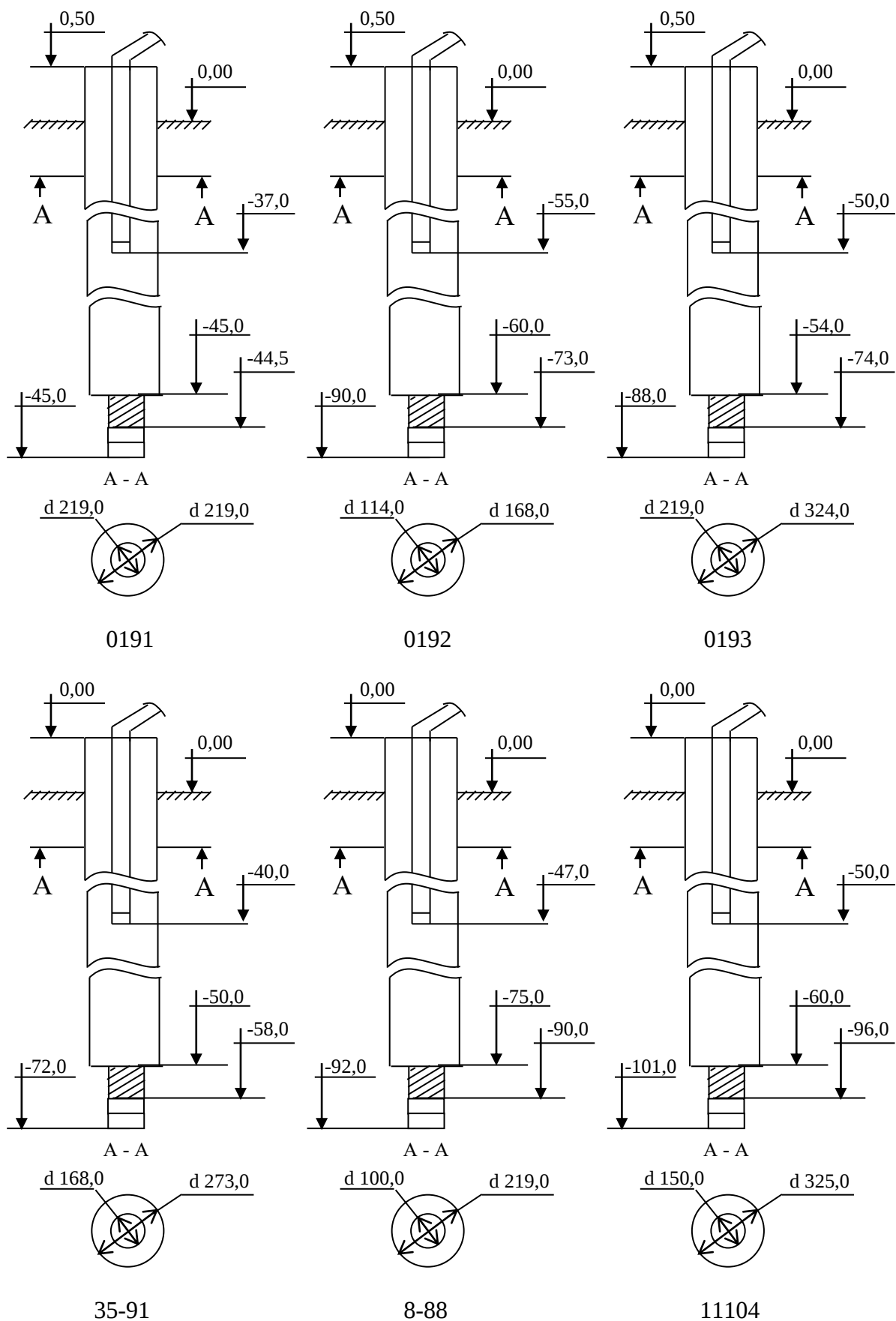
Рисунок 3 – Принципиальная схема установки водоподъемного оборудования в скважинах Ярковского сельсовета
