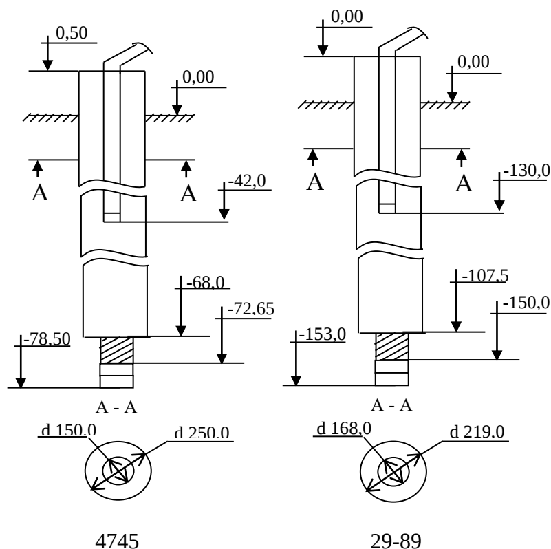
Рисунок 6 – Принципиальная схема установки водоподъемного оборудования в скважинах Ярковского сельсовета
