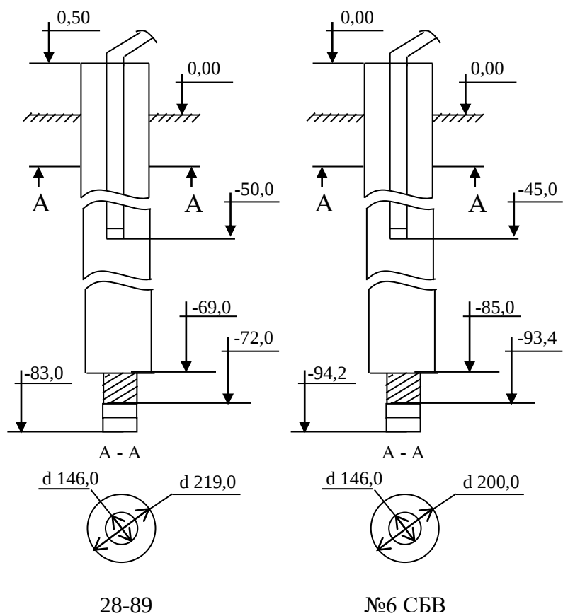
Рисунок 5 – Принципиальная схема установки водоподъемного оборудования в скважинах Ярковского сельсовета
